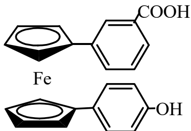
Рис. 2. Строение бис-1-(3-карбоксифенил)-1'-(4-оксифенил)- ферроцена IIa .
