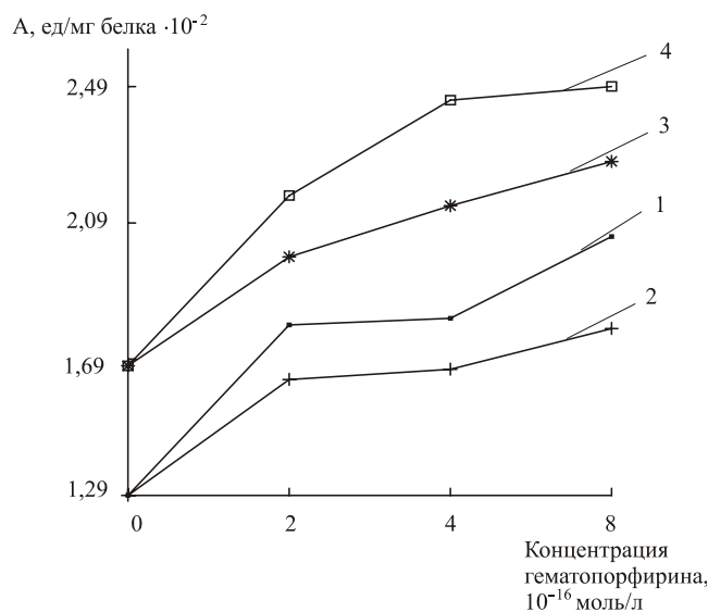
Рис. 2. Активность МПО облученной системы Нф-ГП; 1,3 - в присутствии и 2,4 - после удаления ГП; 3,4 - в присутствии аскорбиновой кислоты. pH реакционной смеси 7,4; доза облучения - 0,6 Дж/см 2 .
