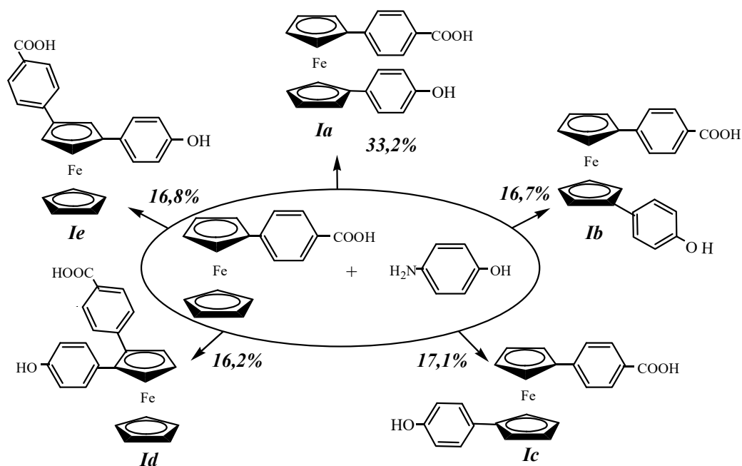
Рис. 1. Возможные изомеры дизамещенных продуктов, образующие в реакции диазотирования пара-ферроценбензойной кислоты с пара-аминофенолом.
