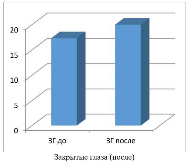
Рис. 2. Изменение средней мощности альфа ритма до и после спелеосанса
