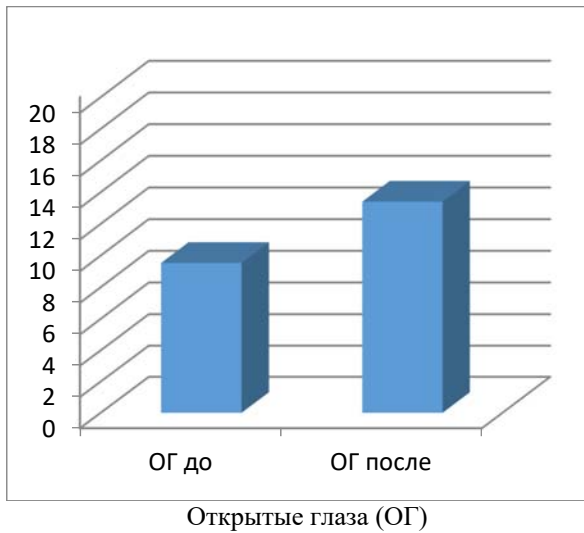
Рис. 2. Изменение средней мощности альфа ритма до и после спелеосанса
