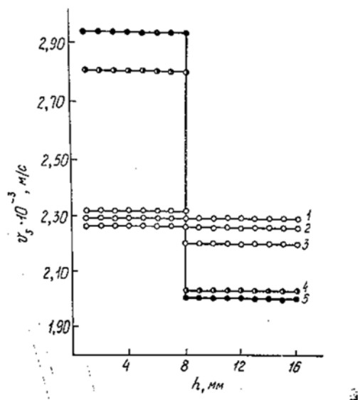
Рис.1. Изменение скорости распространения ультразвука по высоте столба расслаившегося расплава Cu_{82,5}Te_{17,5} при 1513(1), 1485(2), 1478(3), 1425(4), 1398 К (5).
