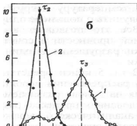
Рис.1. Вариационные диаграммы (а) и кривые распределения (б) долговечности массивных образцов пленки (толщиной 100 мкм) ПММА марки СО-95 при 293 К и различных растягивающих напряжениях (в МПа): 1 - 90 МПа; 2 - 75; 3-60; 4- 40; 5 - 35
