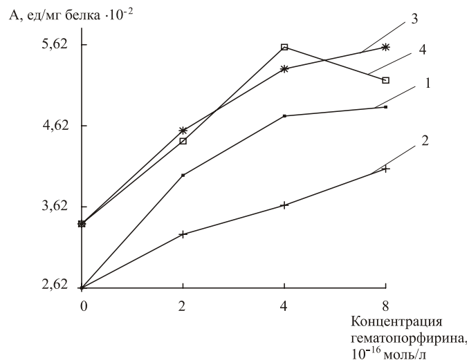
Рис. 1. Активность МПО облученной системы Нф-ГП; 1,3 - в присутствии и 2,4 - после удаления ГП; 3,4 - в присутствии аскорбиновой кислоты. pH реакционной смеси 6,0; доза облучения - 0,6 Дж/см 2 .
