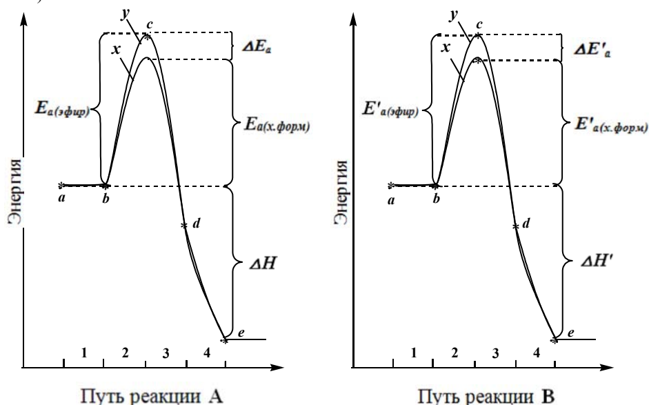
Рис 2. Схема TS перехода реакций диазотирования пара- и метаферроценилбензойных кислот с пара-аминофенолом. Где x и y – переходные состояния реакций в среде хлороформа и диэтилового эфира соответственно; E_{a(эфир)}=2,689\text{кЖ/моль} ; E_{a(х.форм)}=2,648\text{кЖ/моль} ; \Delta E_a=50,6\text{Ж} ; \Delta H=-1,055\text{кЖ/моль} ; E'_{a(эфир)}=2,493\text{кЖ/моль} ; E'_{a(х.форм)}=2,437\text{кЖ/моль} ; \Delta E'_a=56\text{Ж} ; \Delta H'=-1,06\text{кЖ/моль} .
