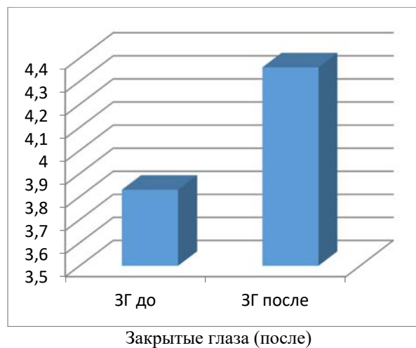
Рис. 4. Изменение средней мощности бета-2 ритма до и после спелеосанса
